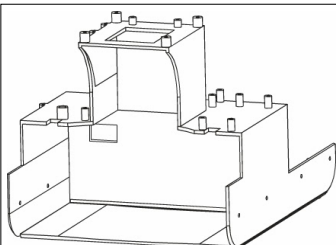
10064661 BASE EP950 REV.2
